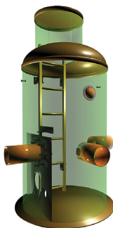
Рис 20. Общий вид «FloTenk-KK».
