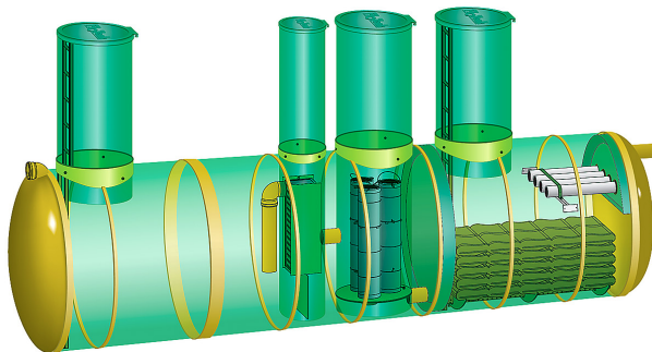
Рис 28. Общий вид (КСО) «FloTenk-OP-OM-SB» (вариант исполнения с губчатым фильтром в маслобензо-отделителе и сорбентом в сорбционном блоке)
