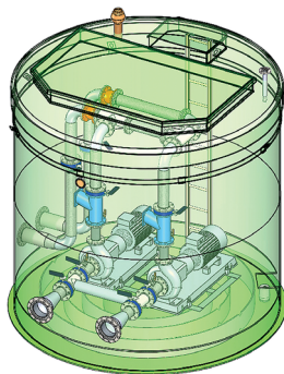
Рис 30. Комплектная насосная станция пожаротушения «FloTenk-PNS», общий вид.
