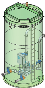
Рис 31. Комплектная насосная станция повышения давления «FloTenk-KNS-DRY», общий вид.
