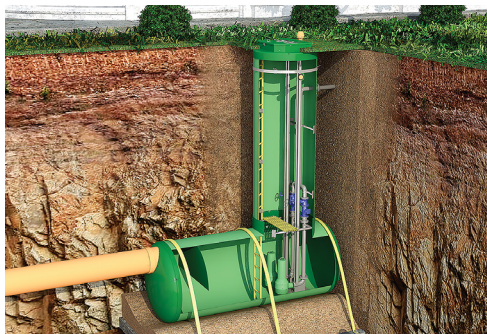
Рис 17. Комплексная насосная станция горизонтального исполнения «FloTenk-KNS-G», общий вид.
